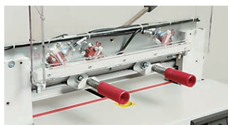
安全に簡単に裁断刃交換が出来る裁断刃交換工具
